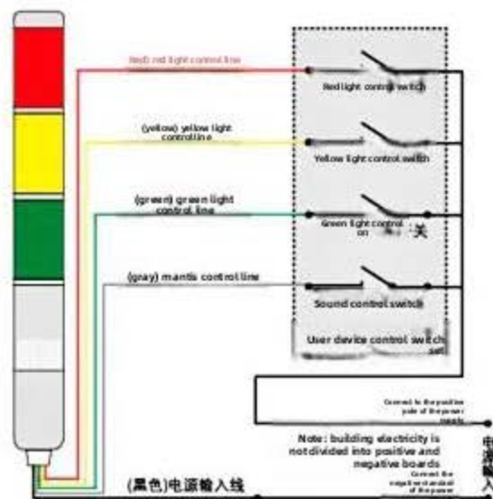
12v/24v wiring diagram
